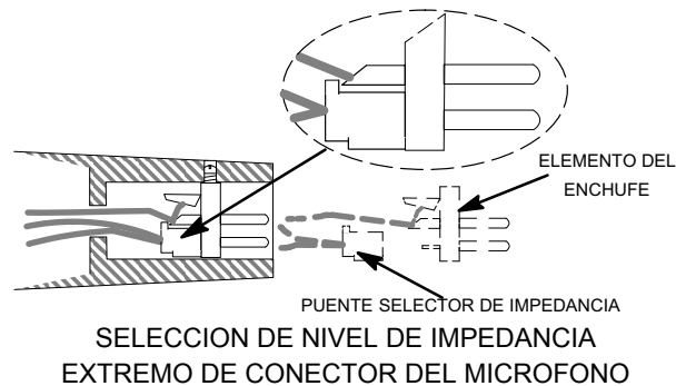
SELECCION DE NIVEL DE IMPEDANCIA EXTREMO DE CONECTOR DEL MICROFONO
