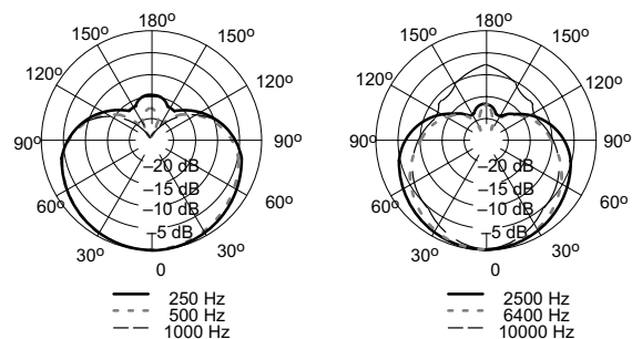
TYPISCHE POLARCHARAKTERISTIK ABBILDUNG 2
