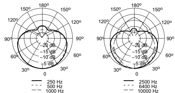
COURBES DE DIRECTIVITÉ TYPIQUES
