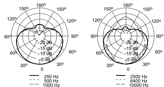
TIPICI DIAGRAMMI POLARI
