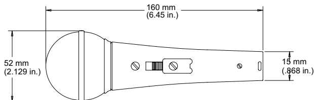
DIMENSIONES TOTALES FIGURA 3
