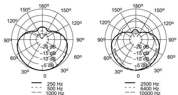
PATRONES DE CAPTACION POLAR TÍPICOS FIGURA 2
