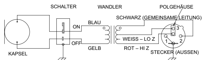
INTERNE ANSCHLÜSSE ABBILDUNG 5
