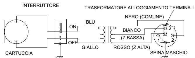
CONNESSIONI INTERNE FIGURA 5
