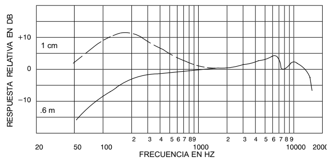
RESPUESTA DE FRECUENCIA TÍPICA FIGURA 1
