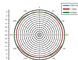
Omni
